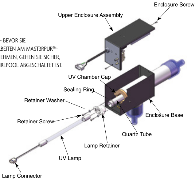
Abbildung 2: Spa Solar Eclipse Explosionsansicht
