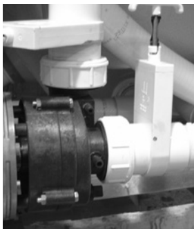
Scheibenventil und Pumpenanschluss
